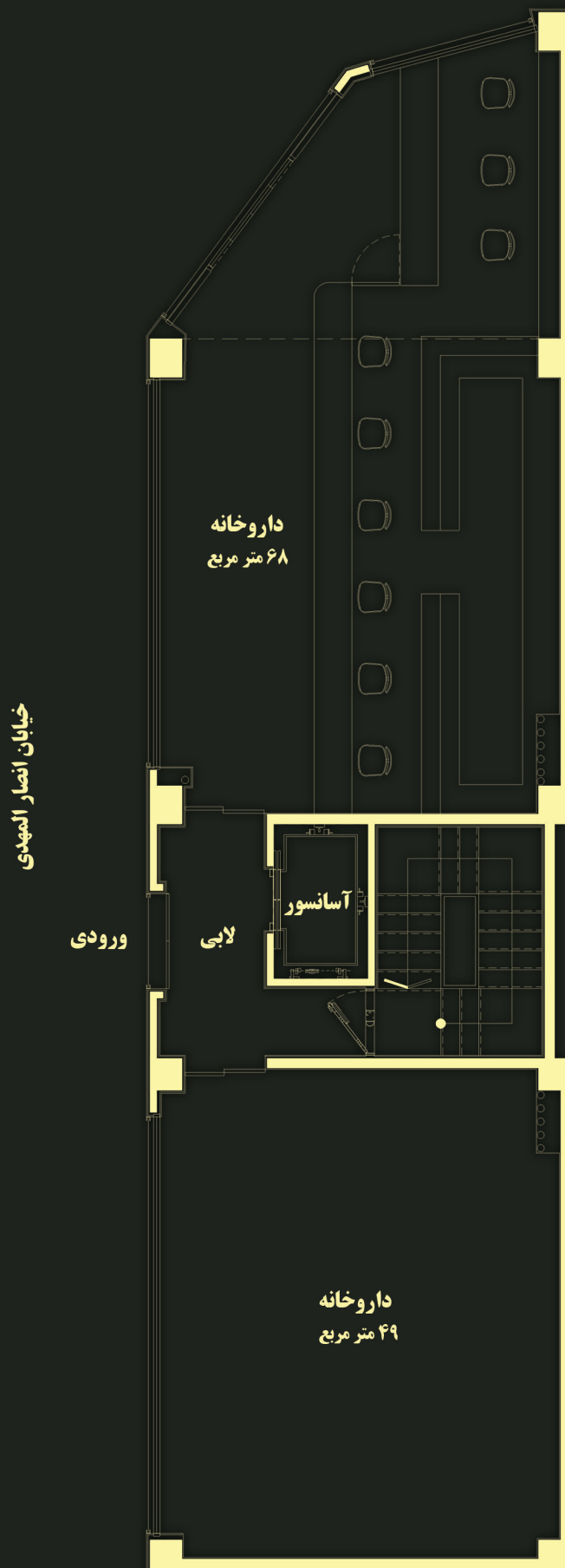
پلان طبقه همکف
