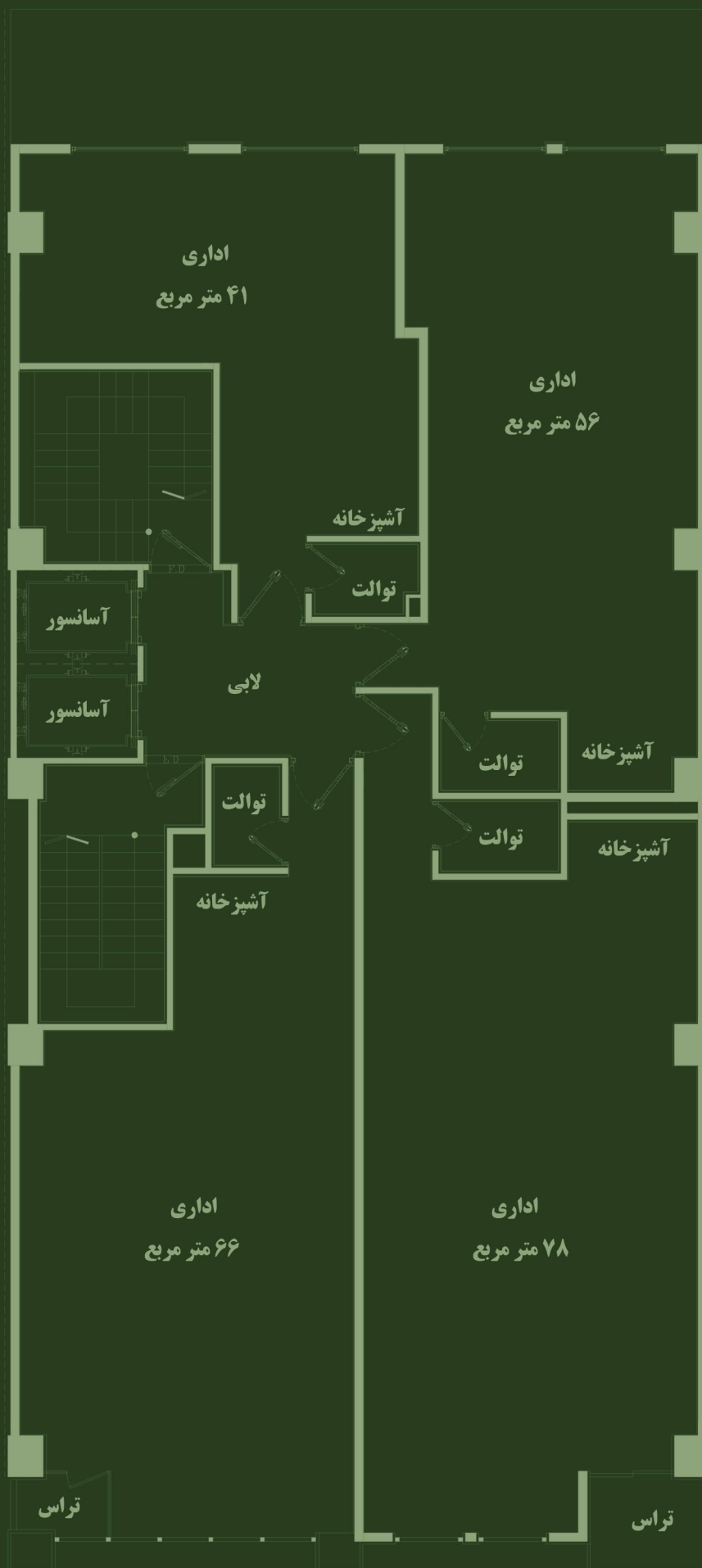
پلان طبقه سوم و چهارم
